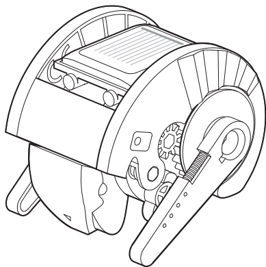
齒輪箱模組 Gear Box Module
