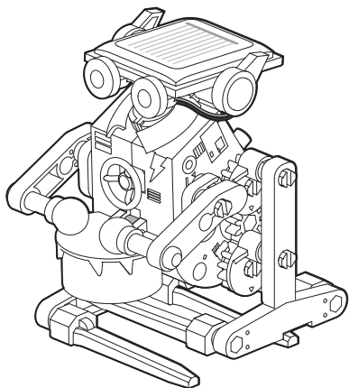
齒輪箱模組 Gear Box Module
