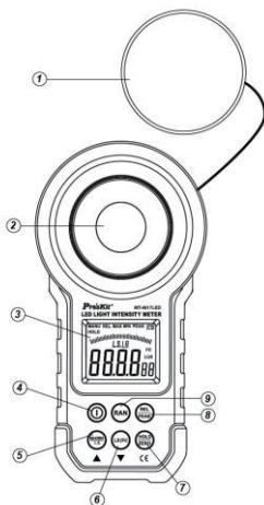
MT-4617 平面圖
