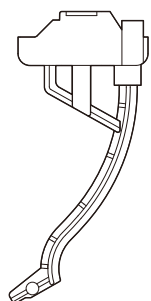
側視圖 Side View
