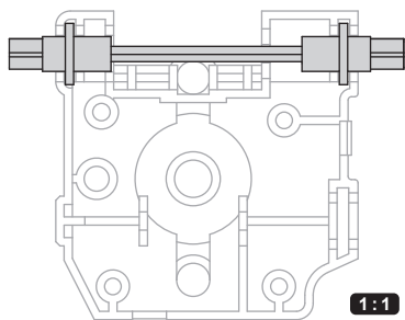
俯視圖 Top View
