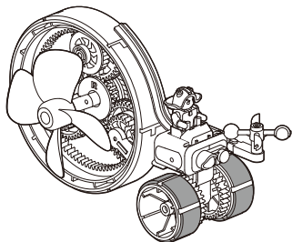
齒輪箱 Gear Box MODULE
