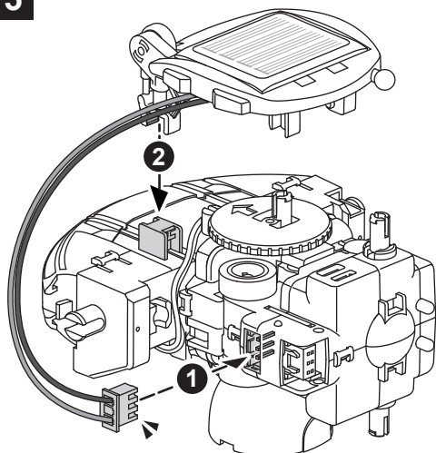
太陽能模組 (組裝見第5頁)
