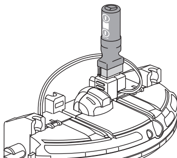
方式2：電池充電
