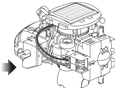
太陽能模組 (組裝見第5頁)
